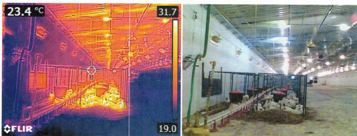
Fot. 1 Obraz z kamery termowizyjnej (po lewej) i standardowo (po prawej)- ogólny wygląd kurnika doświadczalnego
