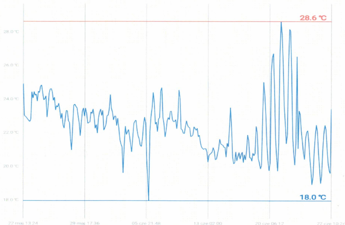
Ryc. 1. Temperatura powietrza w boksach z ptakami w grupie kontrolnej (K) w okresie trwania doświadczenia [°C] - rejestrator Efento
